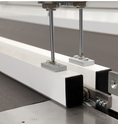
Double press bar (Flexicut)/ Doble prensatelas (Flexicut)
